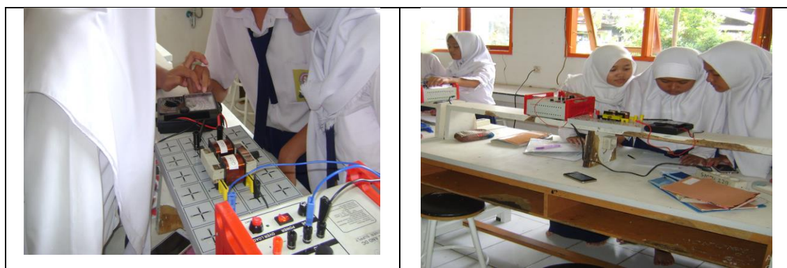
Gambar 3: Aktivitas peserta didik melakukan pengukuran transformator step up
